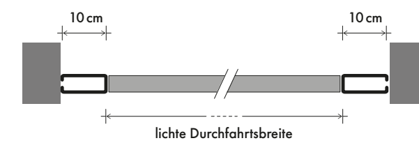
EINBAU ZWISCHEN DER LAIBUNG
