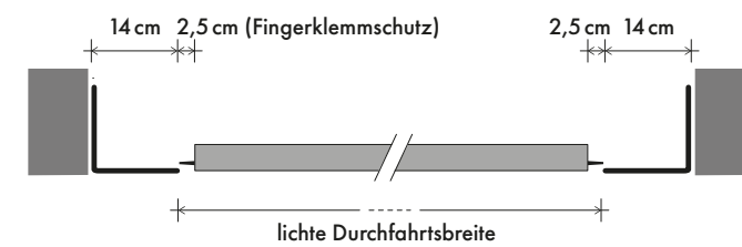
EINBAU ZWISCHEN DER LAIBUNG
