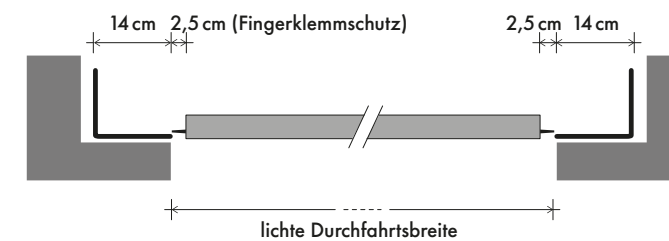
EINBAU HINTER DER LAIBUNG
