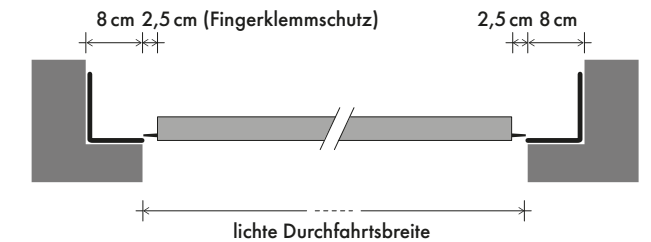
EINBAU HINTER DER LAIBUNG
