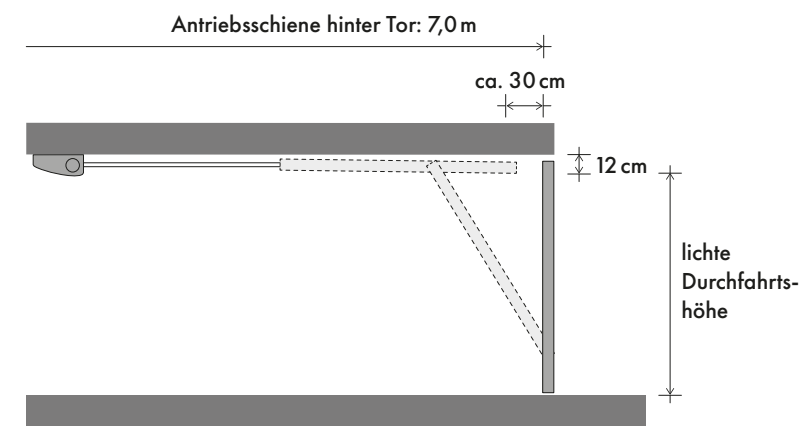
EINBAU UNTER GLATTER DECKE
