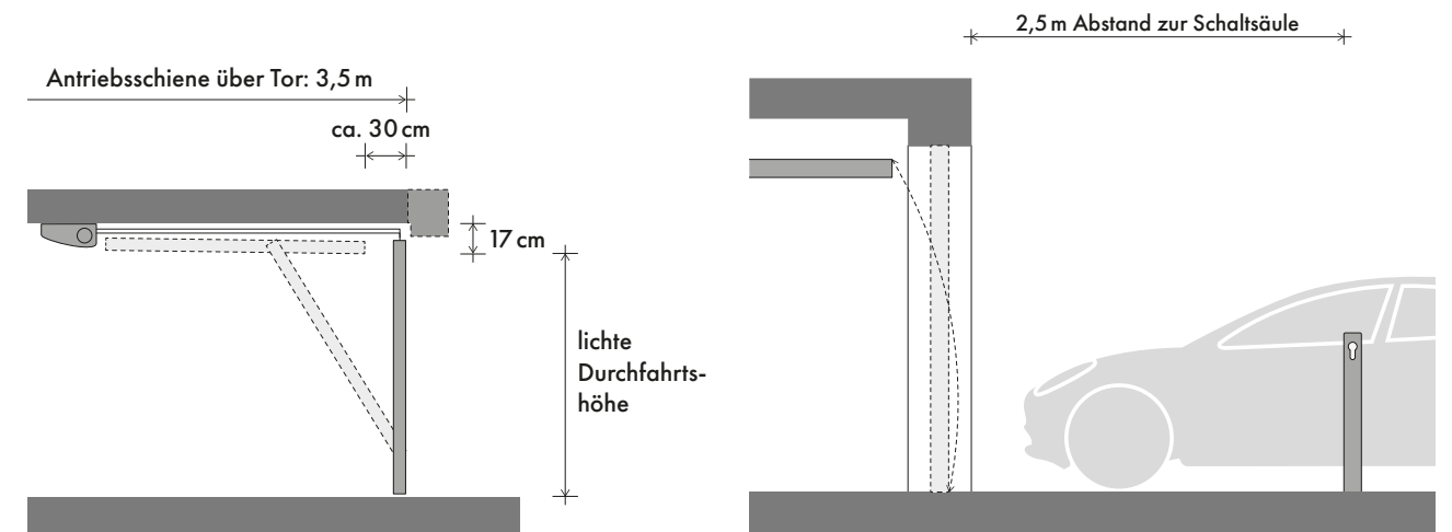
EINBAU HINTER STURZ/ UNTER GLATTER DECKE
